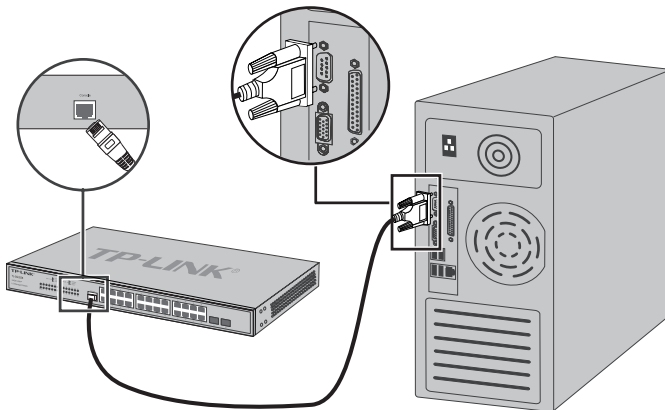
图3-3 Console端口连接示意图
