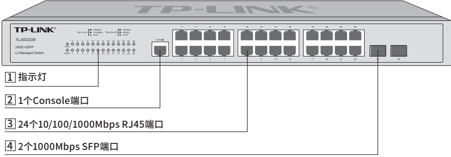
图1-3 TL-SG3226前面板示意图
