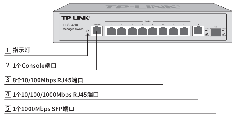
图1-12 TL-SL3210前面板示意图
