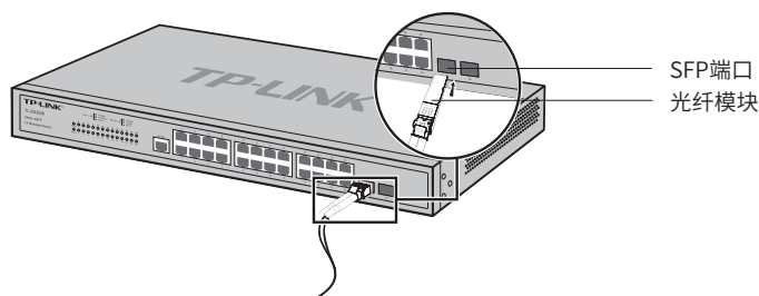
图3-2 SFP端口连接示意图
