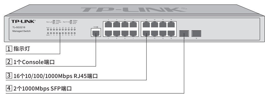
图1-4 TL-SG3218前面板示意图
