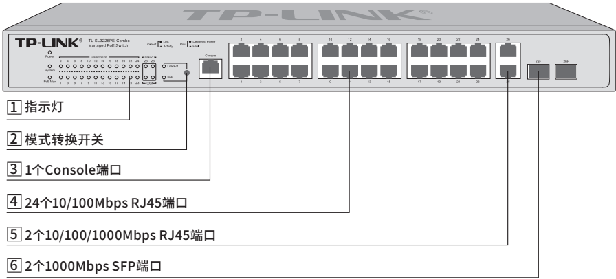
图1-14 TL-SL3226PE-Combo前面板示意图
