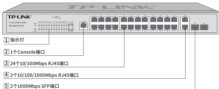
图1-8 TL-SL3226-Combo前面板示意图
