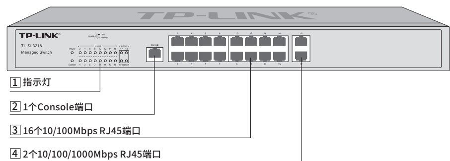
图1-11 TL-SL3218前面板示意图
