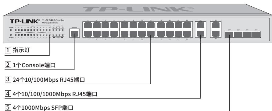
图1-7 TL-SL3428-Combo前面板示意图
