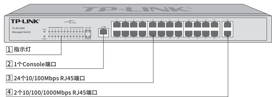
图1-9 TL-SL3226前面板示意图
