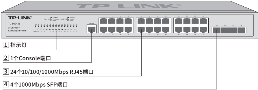
图1-2 TL-SG3428前面板示意图
