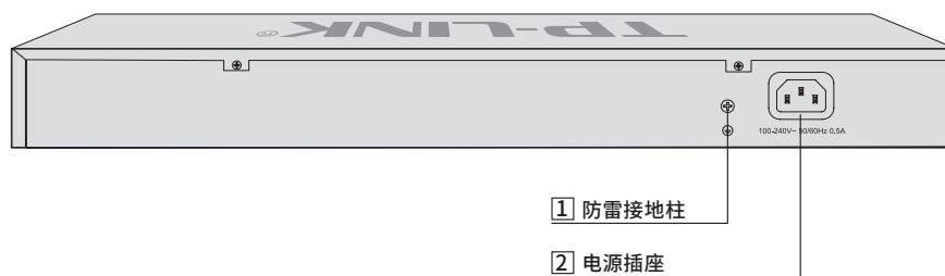
图1-17 后面板示意图
