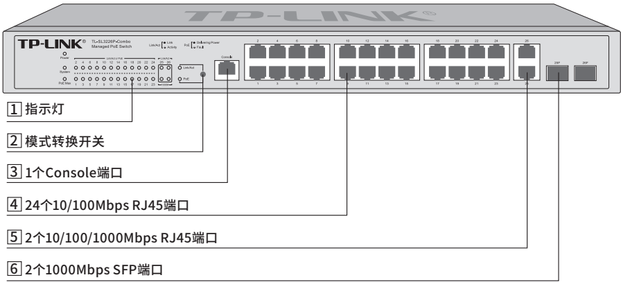
图1-15 TL-SL3226P-Combo前面板示意图
