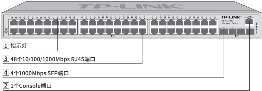
图1-1 TL-SG3452前面板示意图
