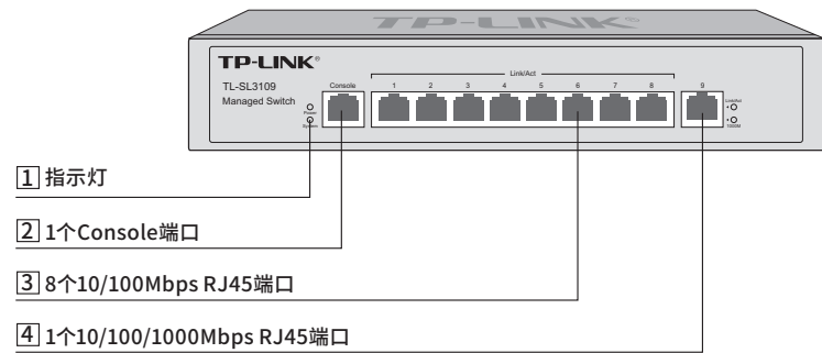
图1-13 TL-SL3109前面板示意图
