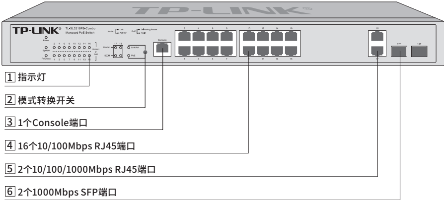
图1-16 TL-SL3218PE-Combo前面板示意图
