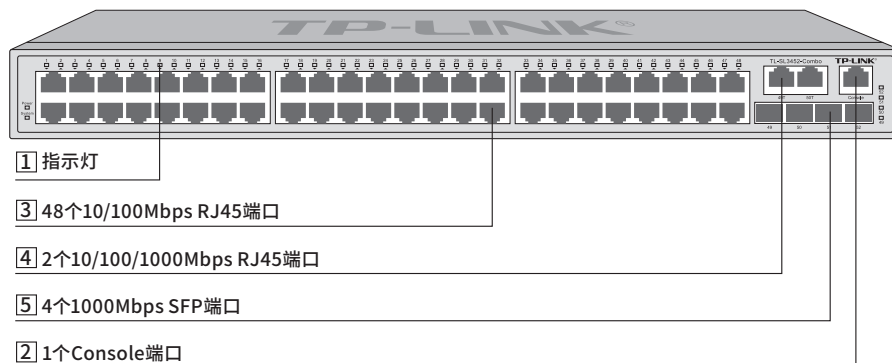
图1-6 TL-SL3452-Combo前面板示意图
