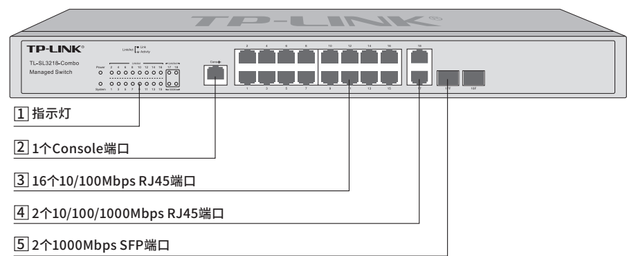
图1-10 TL-SL3218-Combo前面板示意图
