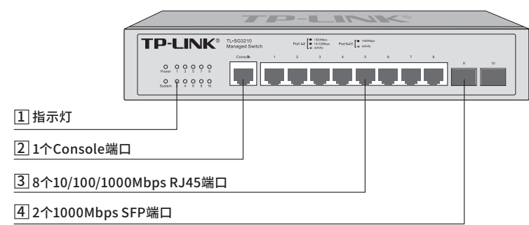
图1-5 TL-SG3210前面板示意图
